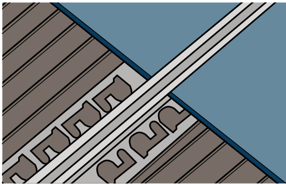
Junta prefabricada
